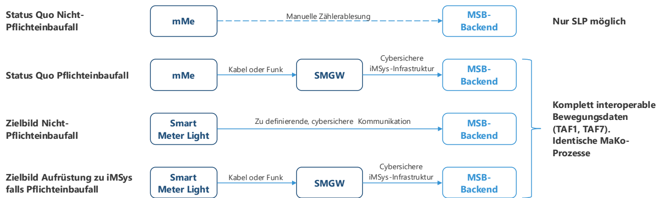
Abbildung 9: Darstellung der unterschiedlichen Konfigurationen im Messwesen bei Einführung eines "Smart Meter Lights". Ab dem MSB Backend sollten alle Systeme wie im Status Quo weiterbetrieben werden können.
