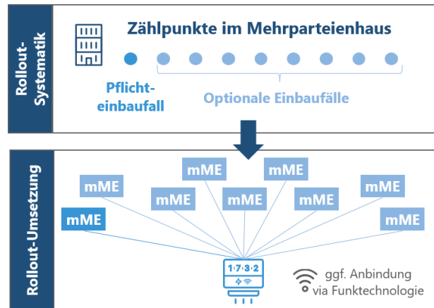
Abbildung 7: Umsetzung der Rolloutsystematik im Mehrparteienhaus
